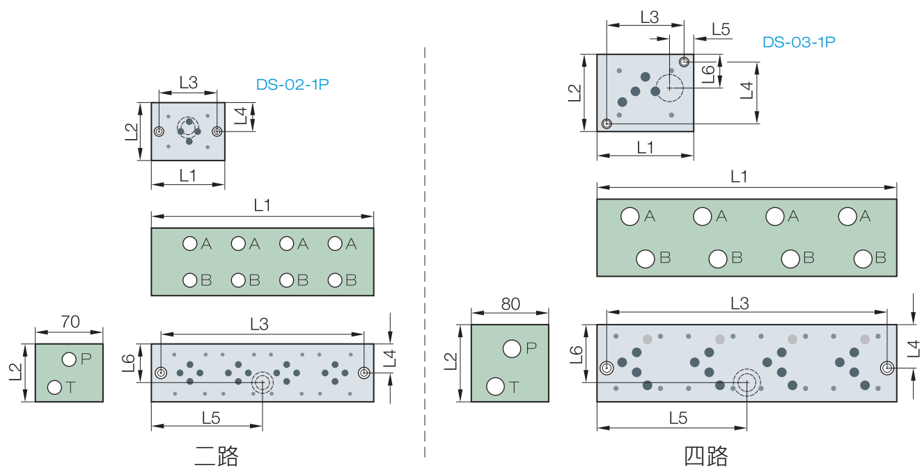
固定孔位置尺寸及迴油孔位置尺寸
